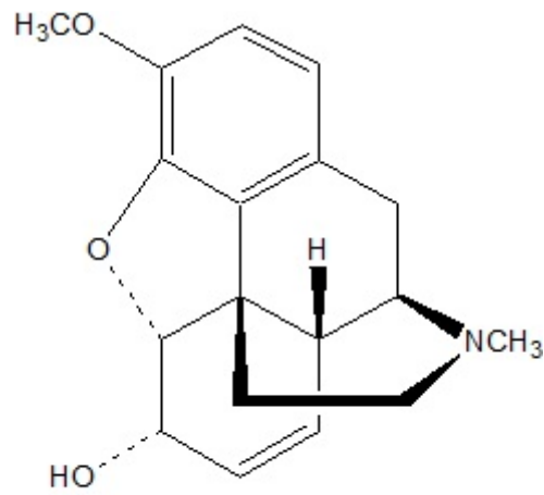
Codeine
